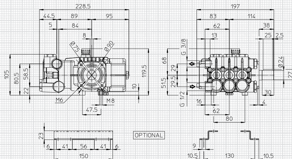
Dimensioni d'ingombro (mm) - Overall Dimensions (mm)
