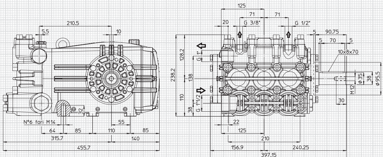
Dimensioni d'ingombro (mm) - Overall Dimensions (mm)
