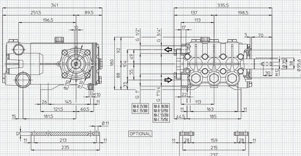
Dimensioni d'ingombro (mm) - Overall Dimensions (mm)
